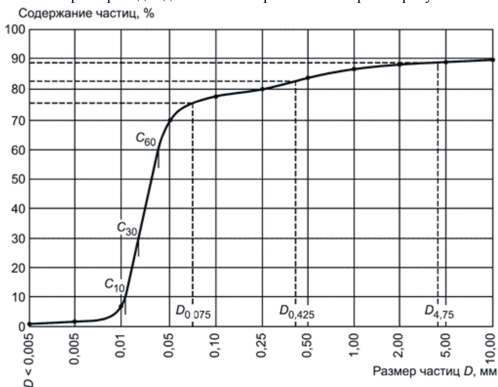
Рисунок Е.2 - Кумулятивная кривая гранулометрического состава
